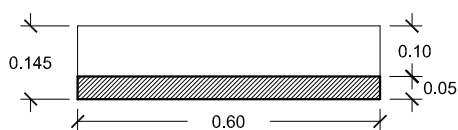
SECCION A-A'
