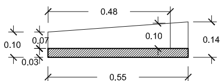
SECCION A-A'
