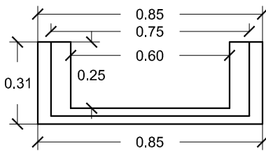
VISTA A
