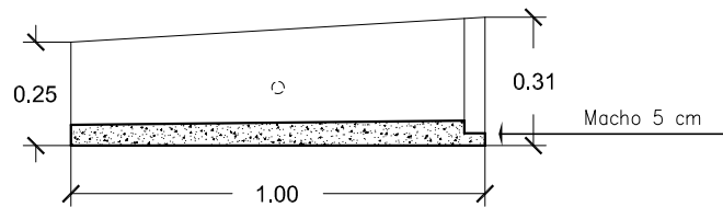
SECCIÓN a-a'
