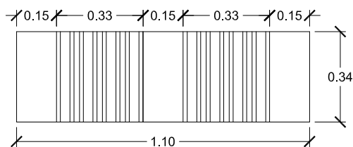
ALZADO
