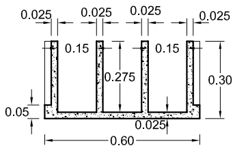
SECCION a-a'
