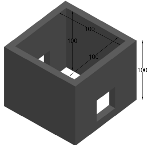
PERSPECTIVA ARQUETA SIN FONDO cotas en cm.
