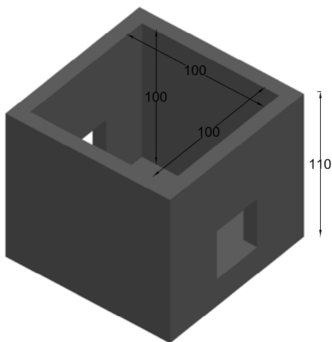
PERSPECTIVA ARQUETA CON FONDO cotas en cm.
