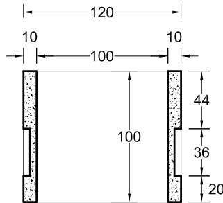
SIN FONDO SECCION a-a'
