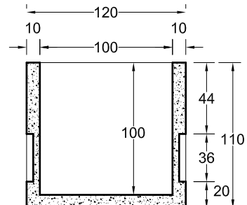
CON FONDO SECCION a-a'
