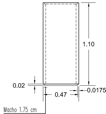
VISTA A
