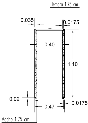
SECCION a-a'
