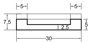
VISTA B
