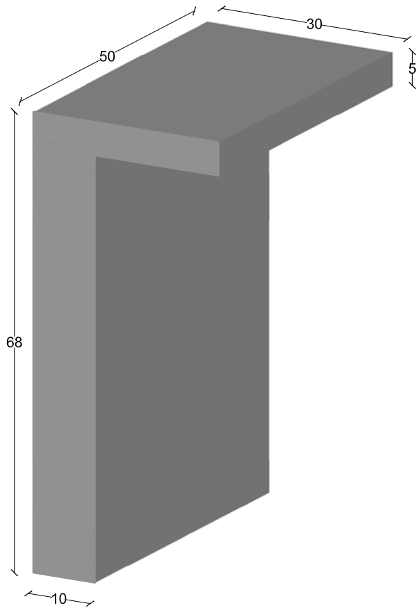
PERSPECTIVA cotas en cm.
