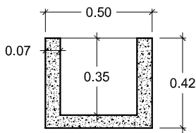
SECCIÓN a-a'
