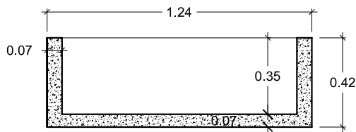
SECCIÓN b-b'
