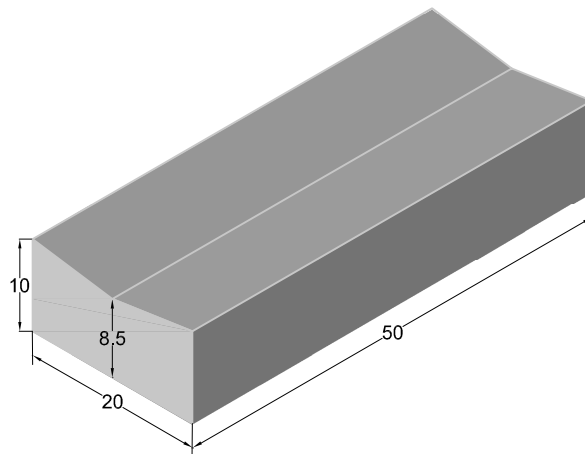
PERSPECTIVA cotas en cm.
