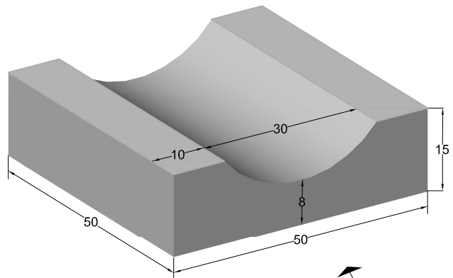
PERSPECTIVA cotas en cm.
