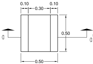
PLANTA SIN RANURAS
