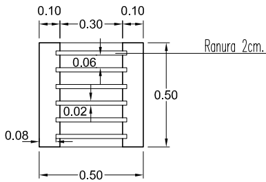
PLANTA CON RANURAS
