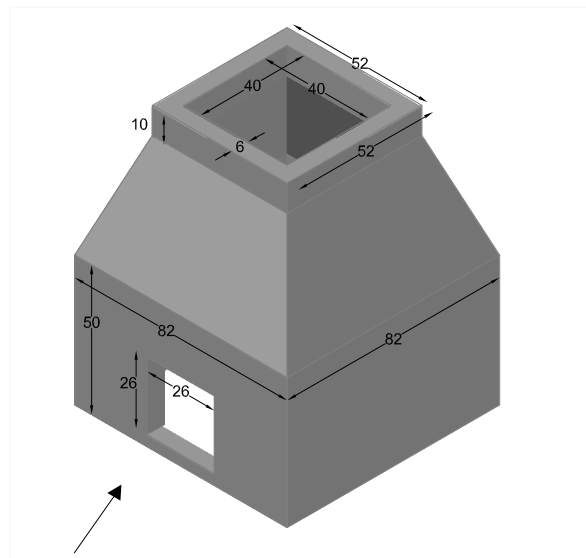
VISTA A
