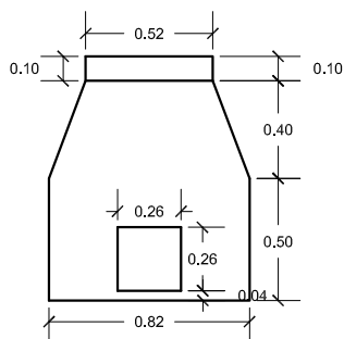
VISTA A
