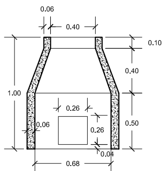
SECCION a-a'
