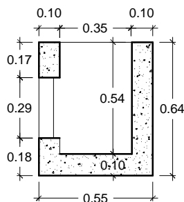
SECCION a-a'
