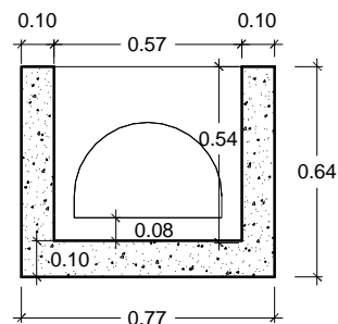
SECCION b-b'
