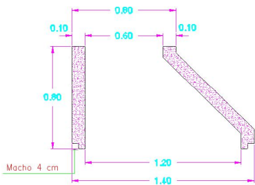
SECCION a-a'
