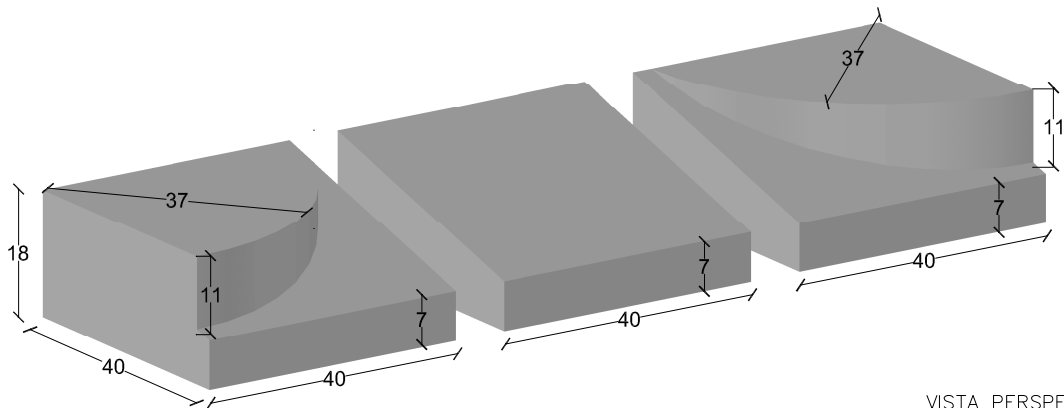
VISTA PERSPECTIVA cotas en cm.
