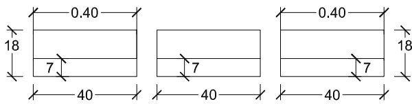
VISTA ALZADO
