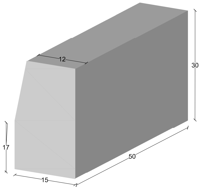
BORDILLO EN MONOCAPA Y BICAPA cotas en cm.
