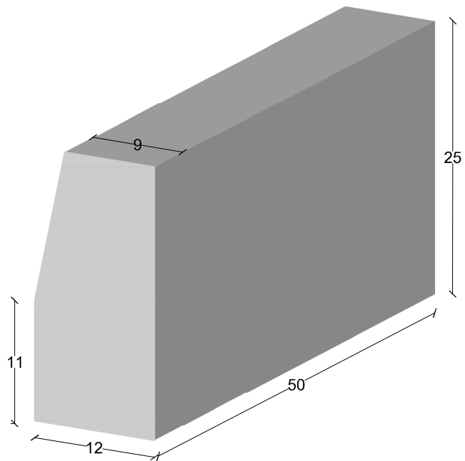
BORDILLO EN MONOCAPA Y BICAPA cotas en cm.
