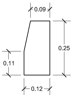
VISTA A
