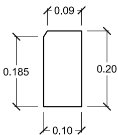
ALZADO
