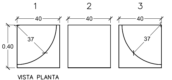
VISTA PLANTA
