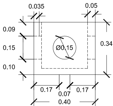
VISTA A
