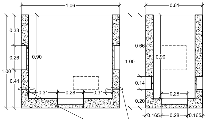
SECCION a-a'
