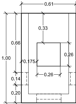
VISTA B
