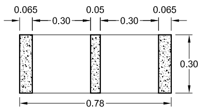
SECCION a-a'
