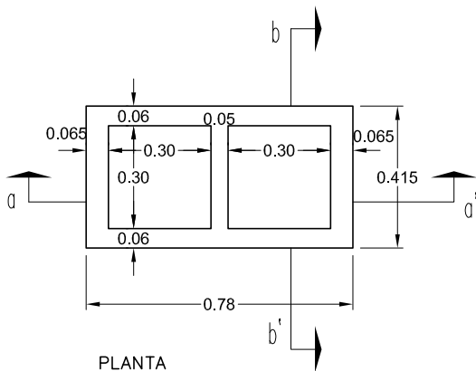
PLANTA
