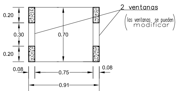
SECCION a-a'
