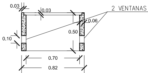
SECCION a-a'
