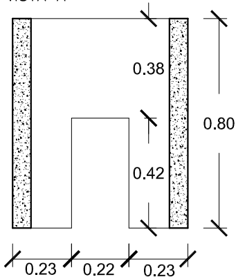
SECCION a-a'
