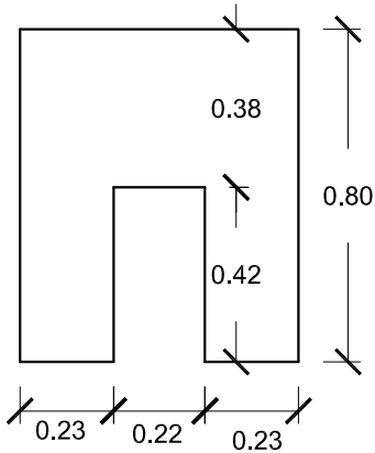
VISTA A
