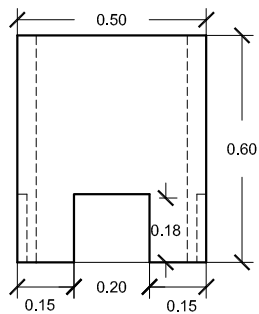
VISTA A
