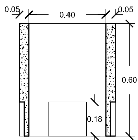
SECCION A-A'
