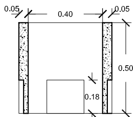
SECCION A-A'
