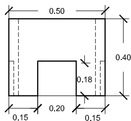
VISTA A
