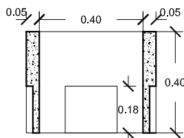
SECCION A-A'
