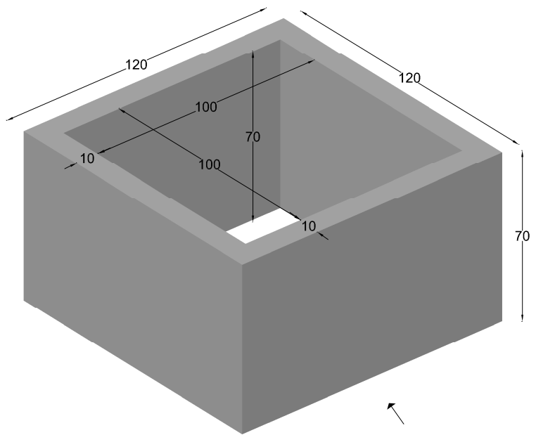
VISTA A
