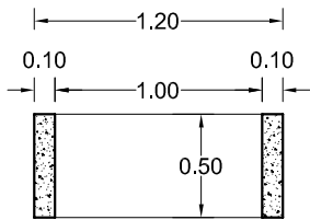
SECCION a-a'
