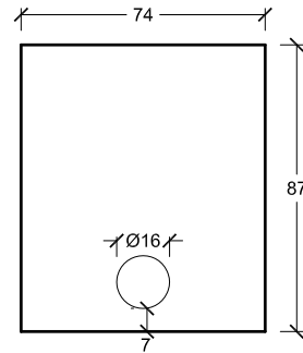
VISTA A
