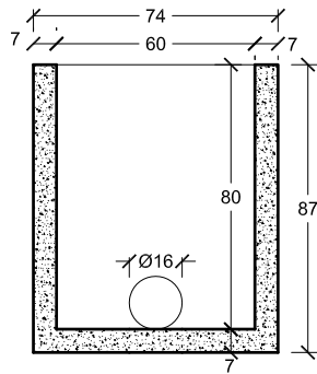
SECCION a-a'
