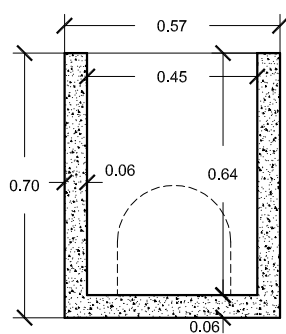
SECCION A-A'
