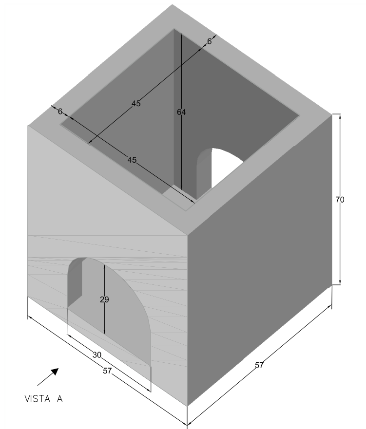
PERSPECTIVA cotas en cm.
