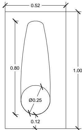
VISTA B
