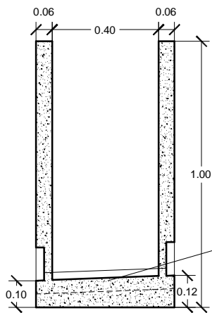
SECCION a-a'
