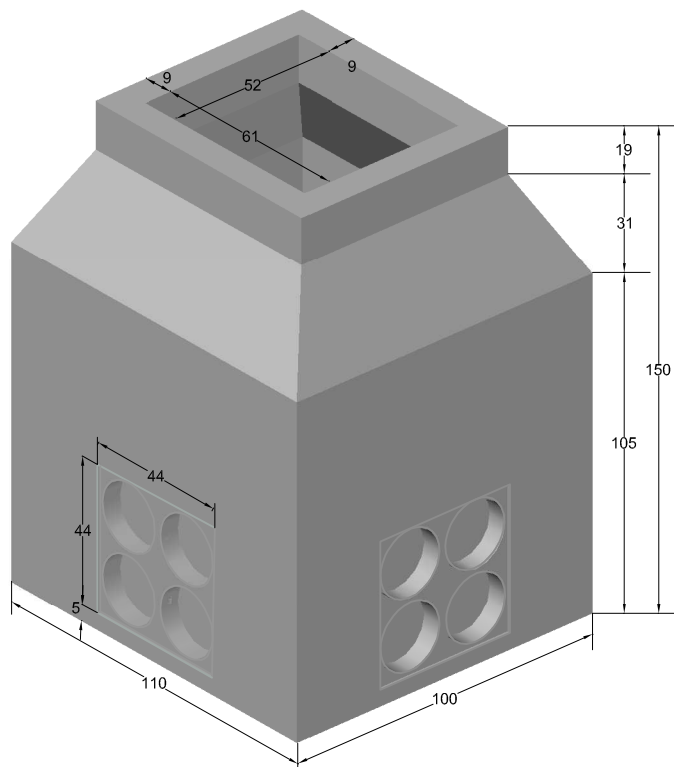
PERSPECTIVA cotas en cm.
