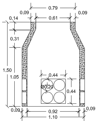
SECCION B-B'
