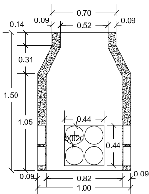
SECCION A-A'
