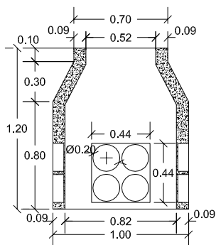
SECCION A-A'
