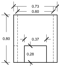
VISTA LATERAL A
