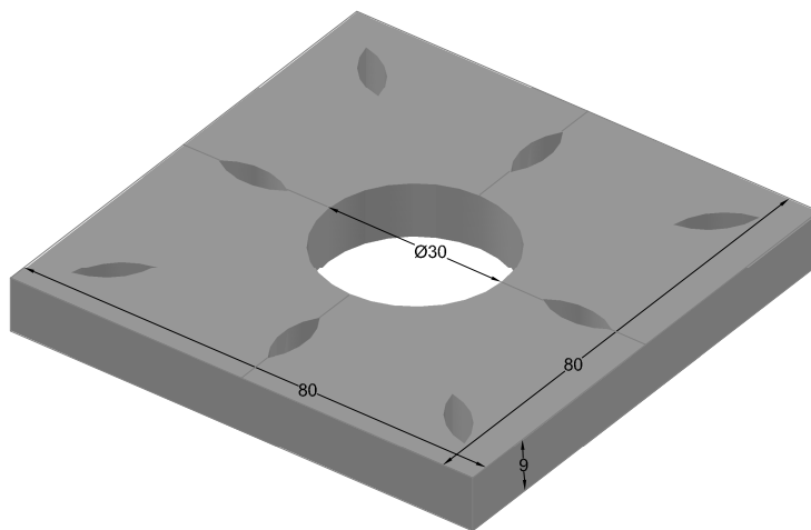
PERSPECTIVA cotas en cm.
